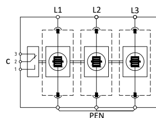
Принципиальная схема
