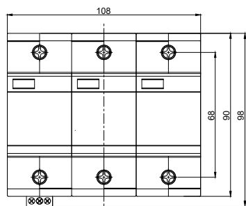
Габаритные размеры
